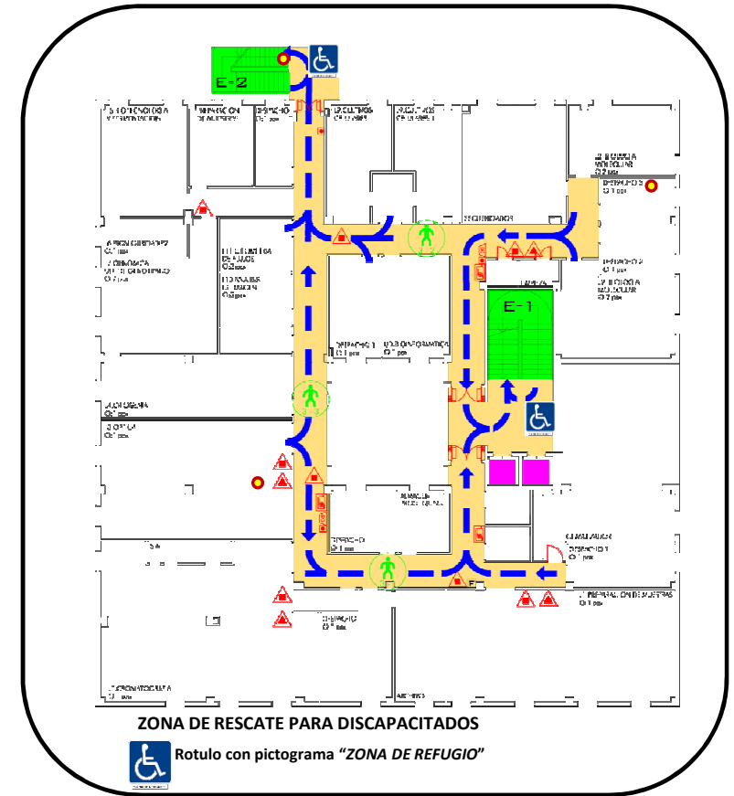
PLANTA TERCERA
