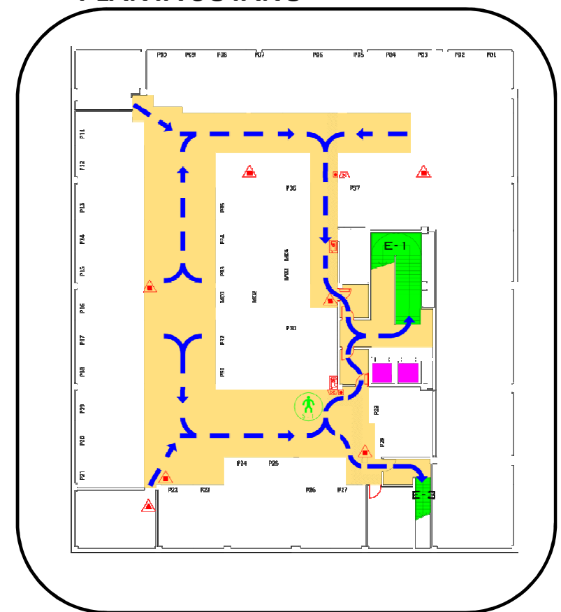
PLANTA SOTANO
